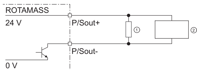
図 24: アクティブパルス出力接続 P/Sout の接続図
