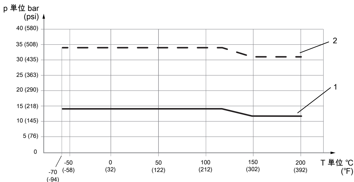
図 11: 流体温度と許容プロセス圧力の関係
