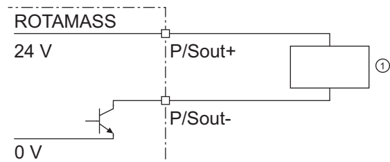
図 29: アクティブステータス出力接続 P/Sout
