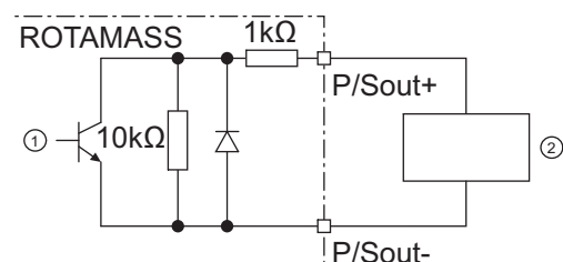
図 33: スイッチングアンプが接続された場合のパッシブパルス出力またはステータス出力
