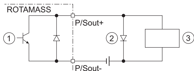
図 28: 機械式カウンタの場合のパッシブパルス出力 P/Sout の接続図
