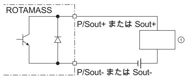
図 31: パッシブステータス出力接続 P/Sout または Sout
