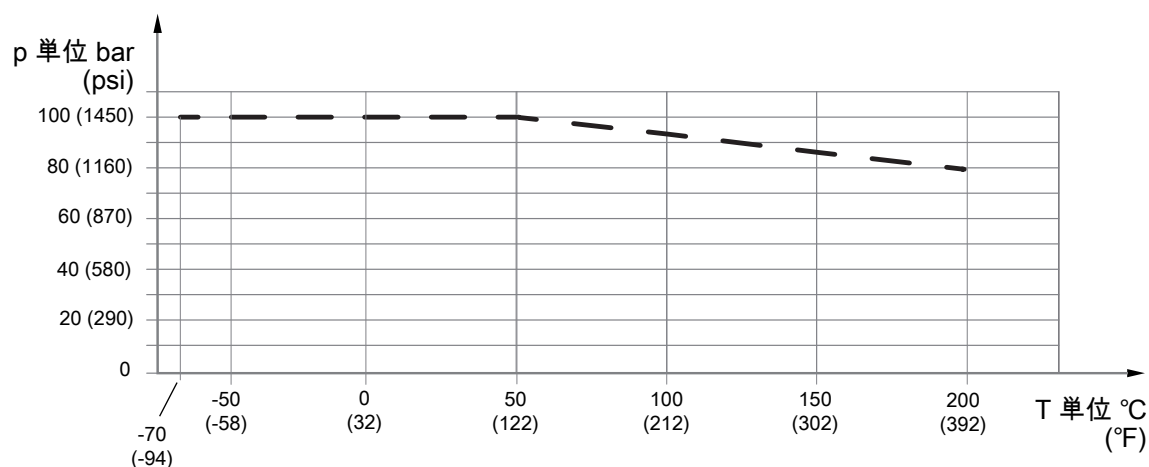
図 10: 流体温度と許容プロセス圧力の関係 (EN 1092-1 PN100 準拠フランジ)
