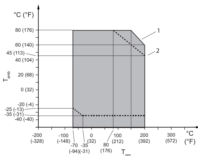
図 14: 許容される流体温度および周囲温度 (分離形)
