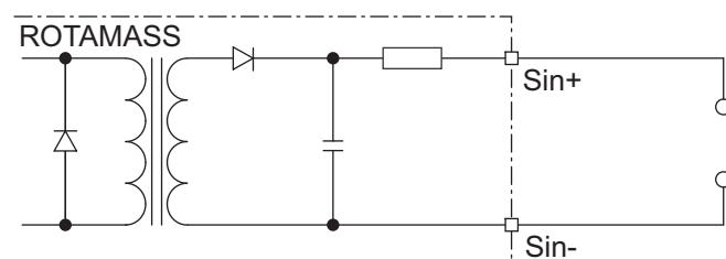
図 34: ステータス入力接続図
