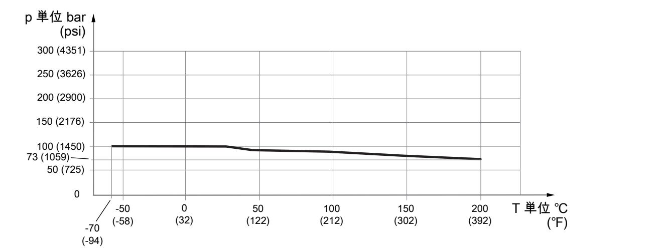
図 12: 流体温度と許容プロセス圧力の関係
