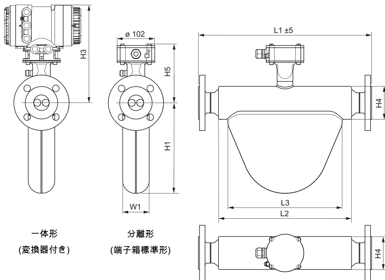
図 16: 寸法 (単位 mm)
