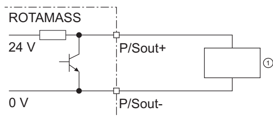
図 26: 内部プルアップ抵抗付き アクティブパルス出力 P/Sout
