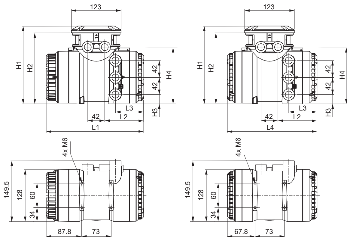
図 17: 変換器の寸法, 単位 mm, (左側: 表示器付き変換器, 右側: 表示器のない変換器)
