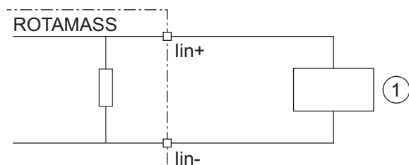
図 23: アクティブ電流出力をもつ外部機器との接続図
