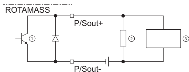
図 27: 電子式カウンタの場合のパッシブパルス出力 P/Sout の接続図
