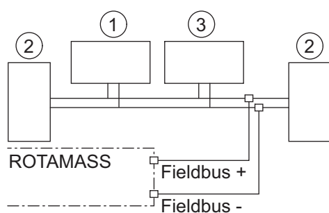
図 36: FOUNDATION Fieldbus 接続図
