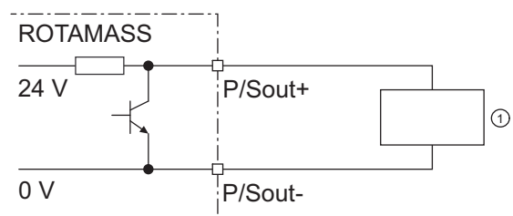
図 30: 内部プルアップ抵抗付き アクティブステータス出力 P/Sout
