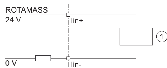
図 22: パッシブ電流出力をもつ外部機器との接続図
