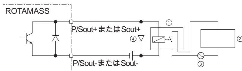
図 32: ソレノイドバルブ回路がある場合のパッシブステータス出力接続 P/Sout または Sout の接続図
