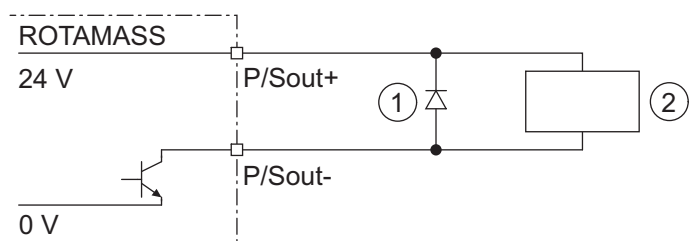
図 25: アクティブパルス出力接続 P/Sout の機械式カウンタとの接続図
