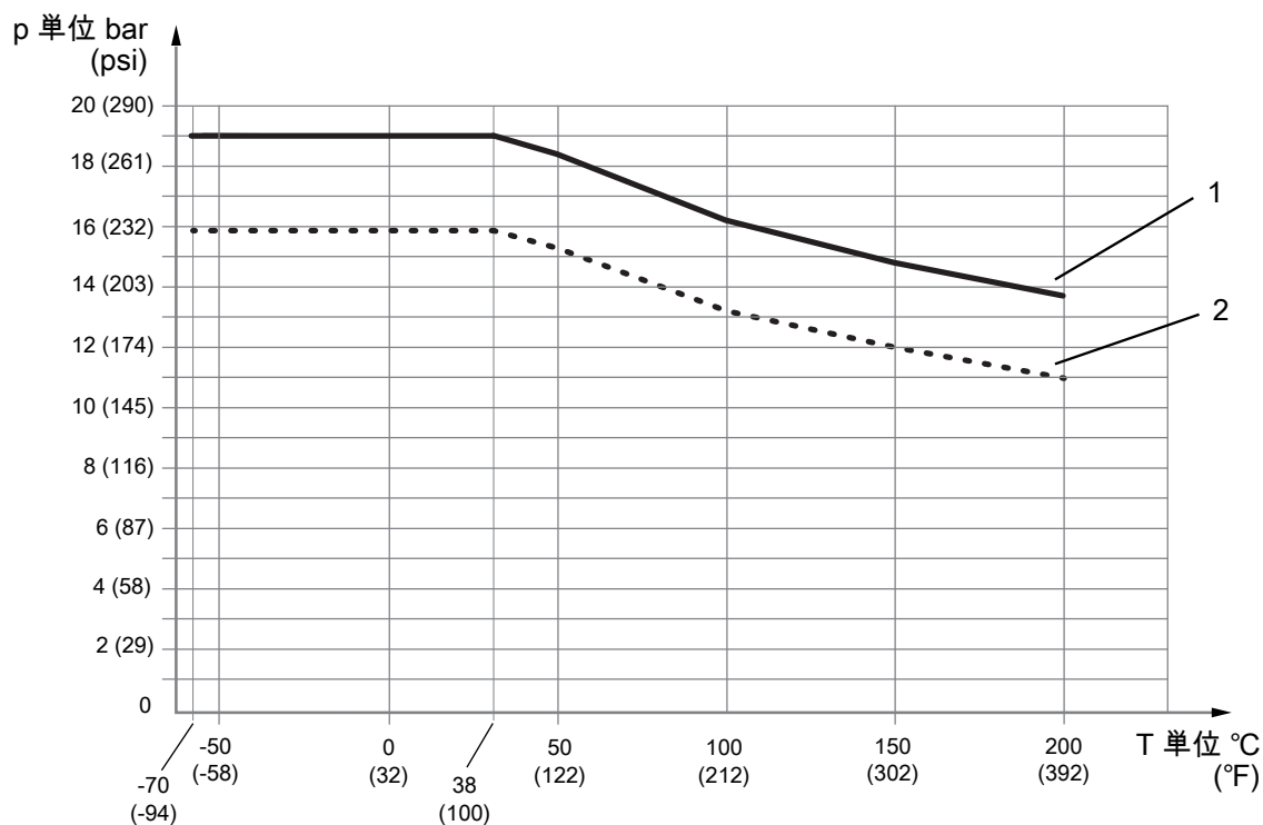
図 7: プロセス接続部の温度と許容プロセス圧力の関係
