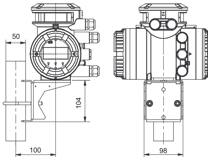
図 18: 変換器の寸法, 単位 mm, (U字金具に取り付け)
