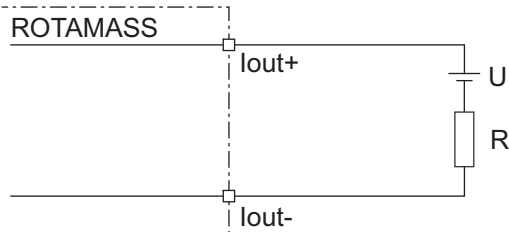
図 21: パッシブ電流出力接続 lout の接続図
